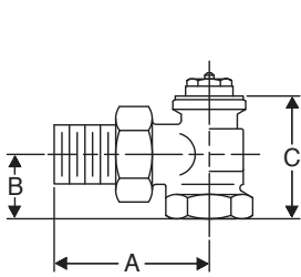
RV-4 Angle
